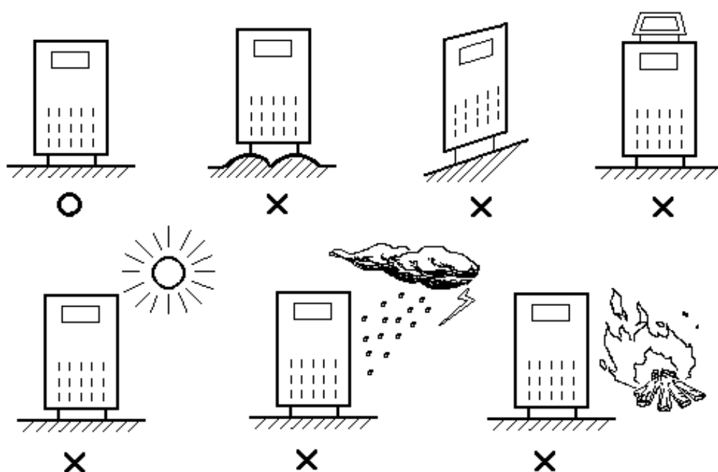
Рис 3.1 Установка ИБП
